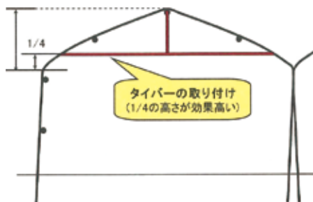
タイバー (はり) の設置
